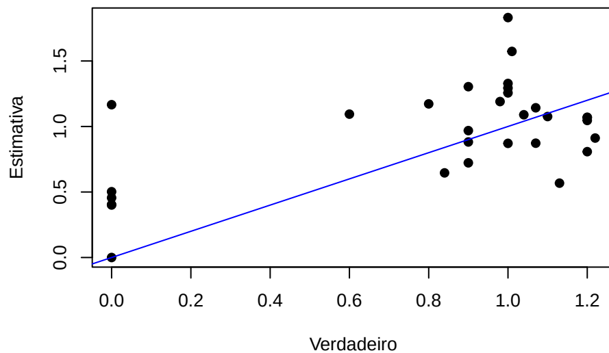
Discriminacao a2
