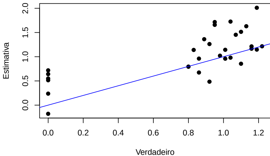
Discriminacao a1
